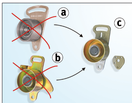
Figure 1: Schema della sostituzione
