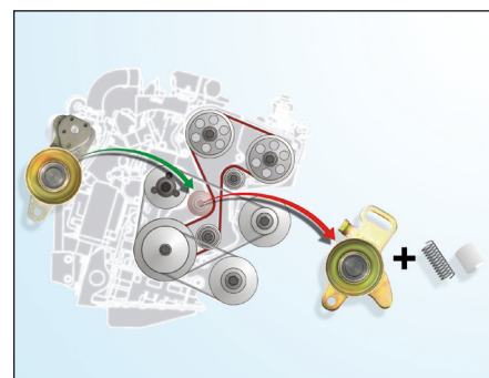
Figure 2: Schema complessivo dell'azionamento
