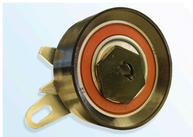
Фигура 1: 531 0342 30
