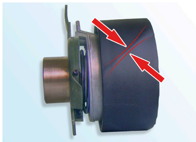
Figura 2: 531 0564 30 (vedere laterală)
