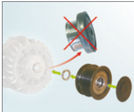
Fig. 2: Montageoverzicht
