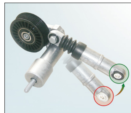
Image 2: versions de la réf. 534 0014 10 avec œillets en plastique blanc et noir sur l'amortisseur hydr.
