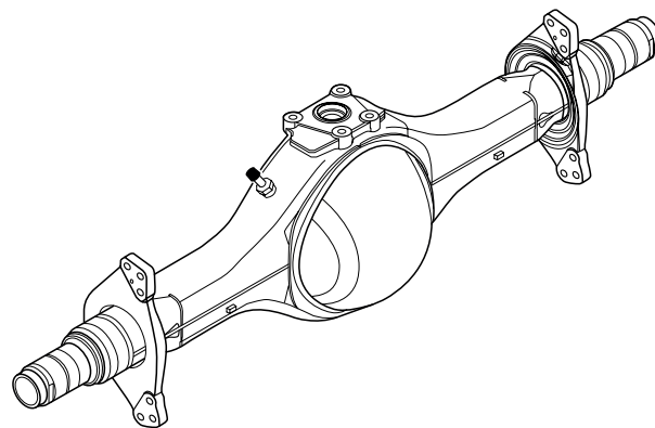
Afbeelding 1: Ontluchtingsventiel op een DAF CF- of XF-as
