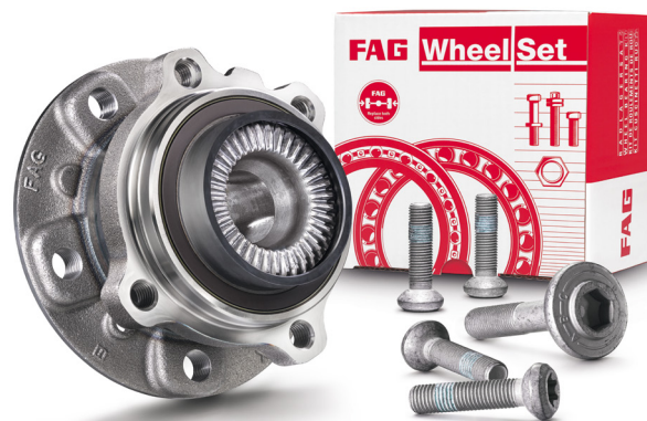
Bild 2: De medlevererade skruvarna skall alltid användas.
