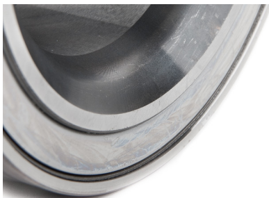
Kuva 3: Truck Hub Unit (pyörän navan laakeriyksikkö) pyörästetyllä reunalla
