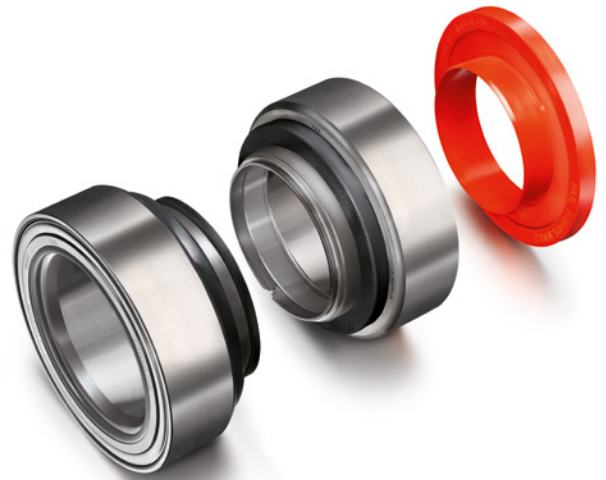
Fig. 1: cuscinetto compatto di ricambio (RIU)
