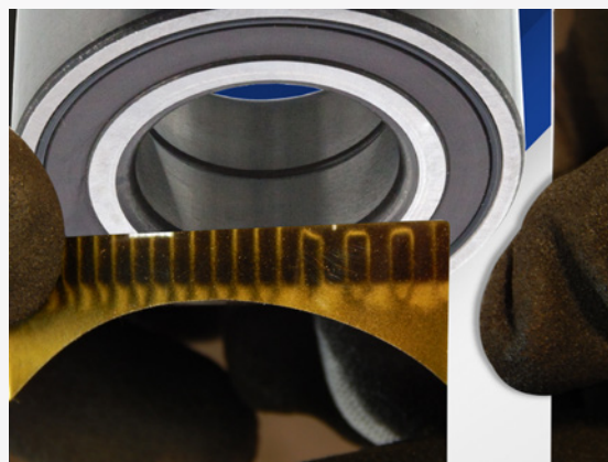
Beispiel eines fehlerhaften Polrads unter Verwendung einer magnetischen Testkarte
