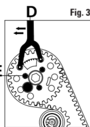
FIGURA 1 Inserire l'apposito attrezzo di bloccaggio dell'albero a camme A. FIGURA 2 Controllare il corretto allineamento della tacca di fasatura verificando che essa sia allineata con l'incisura sul mozzo del pignone dell'albero a camme: B per motori 4 cilindri e C per motori 3 cilindri. FIGURA 3 Inserire l'apposito attrezzo D, per mantenere gli ingranaggi in tensione e serrare le 3 viti E, sfalsate di 120° l'una dall'altra.
