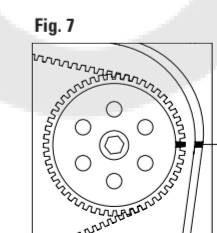
FIGURA 7 Controllare il corretto allineamento delle tacche di fase H (pompa Bosch). FIGURA 8 Controllare il corretto allineamento della tacca di fase I (pompa Lucas).
