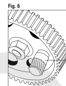
FIGURA 6 Inserire l'apposito attrezzo di bloccaggio della puleggia della pompa di iniezione H. FIGURA 7 Inserire l'apposito attrezzo di bloccaggio della puleggia della pompa di iniezione I.
