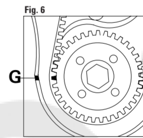
FIGURA 6 Controllare il corretto allineamento delle tacche di fase G. FIGURA 7 Inserire l'apposito attrezzo di bloccaggio del volano H.
