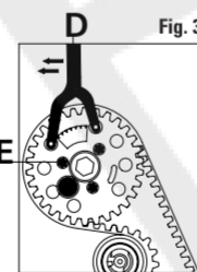
FIGURA 1 Inserire l'apposito attrezzo di bloccaggio dell'albero a camme A. FIGURA 2 Controllare il corretto allineamento della tacca di fasatura verificando che essa sia allineata con l'incavo sul mozzo del pignone dell'albero a camme: B per motori 4 cilindri e C per motori 3 cilindri. FIGURA 3 Inserire l'apposito attrezzo D, per mantenere gli ingranaggi in tensione e serrare le 3 viti E, sfalsate di 120° l'una dall'altra.
