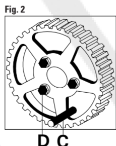
FIGURA 1 Insertar la herramienta especial de inmovilización de árbol de levas A. Los tornillos B, espaciados 120° entre sí, no deben estar situados en las extremidades de las acanaladuras. FIGURA 2 Insertar la herramienta especial de inmovilización de árbol de levas C. Los tornillos D, espaciados 120° entre sí, no deben estar situados en las extremos de las acanaladuras.
