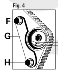
FIGURA 4 Extraer el tornillo F del cárter anterior e insertar la herramienta específica para tensado de correas G, actuando en el punto indicado H hasta lograr alinear el indicador I del tensor de correa con la marca L.
