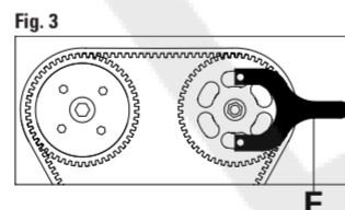
FIGURA 1 Inserire l'apposito attrezzo di comparazione A, sul cilindro N° 1. FIGURA 2 Inserire l'apposito strumento di bloccaggio degli alberi a camme B e verificare il perfetto allineamento delle tacche di fase C e D. FIGURA 3 Attrezzo di mantenimento della tensione degli alberi a camme E.
