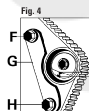
FIGURA 4 Smontare il bullone F del carter anteriore ed inserire l'apposito attrezzo di tensionamento G. Agendo nel punto indicato H, allineare l'indicatore I del tendicinghia con la tacca L.
