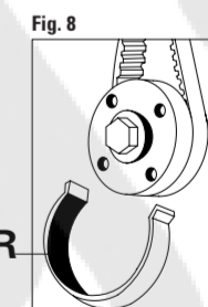
FIGURA 6 Inserire l'apposito attrezzo di bloccaggio del volano P. FIGURA 7 Controllare il corretto allineamento della tacca di fase Q. FIGURA 8 Inserire l'apposito attrezzo di bloccaggio della cinghia di distribuzione R.
