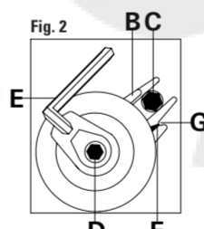
FIGURA 2 Assicurarsi che la piastra B sia fissata al di sotto del bullone di bloccaggio C; allentare il bullone di blocco D e ruotare in senso orario il tendicinghia utilizzando la chiave esagonale E sull'eccentrico di registro; allineare l'indicatore F con la tacca G e serrare, quindi, il bullone di bloccaggio D.
