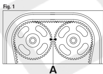
FIGURA 1 Controllare il corretto allineamento delle tacche di fase A.
