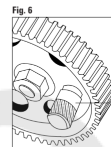
FIGURA 6 Inserire l'apposito attrezzo di bloccaggio della puleggia della pompa di iniezione H. FIGURA 7 Inserire l'apposito attrezzo di bloccaggio della puleggia della pompa di iniezione I.
