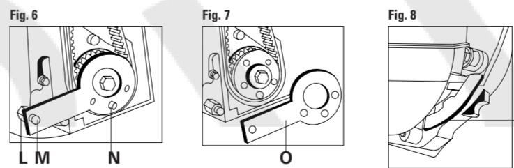
FIGURA 6 Smontare il bullone della pompa dell'olio L e installare al suo posto il prigioniero dell'attrezzo di bloccaggio M. Ruotare l'albero motore fino al PMS del cilindro N°1 e verificare il corretto posizionamento del grano della puleggia dell'albero motore N.
