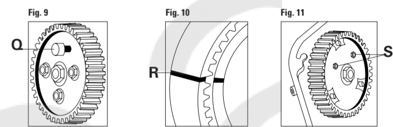
FIGURA 9 Inserire l'apposito attrezzo di bloccaggio della puleggia della pompa di iniezione Q.
