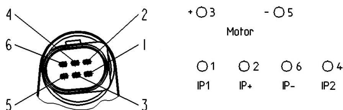
2 - Anschluss / Connector
