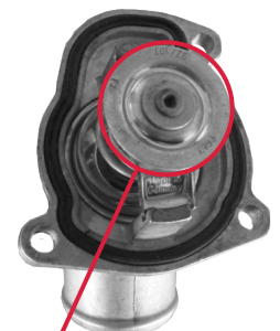
Termostater på eftermarknaden som inte uppfyller OE-specifikationerna. (diameter: >23 mm)
