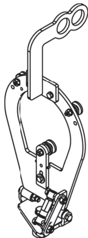
Obr. 1: Montážny prípravok s nosným strmeňom cDISK Blitz Rotary obj. č. 3745410
