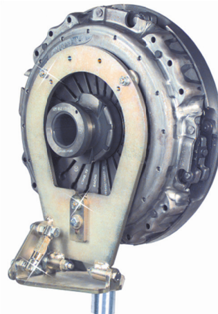
Obr. 3: Montážny prípravok pre prítlačný kotúč Blitz Rotary obj. č. 101758
