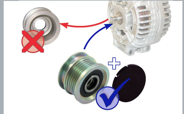
Bild 1: Wechsel von starrer Riemenscheibe auf einen Generatorfreilauf
