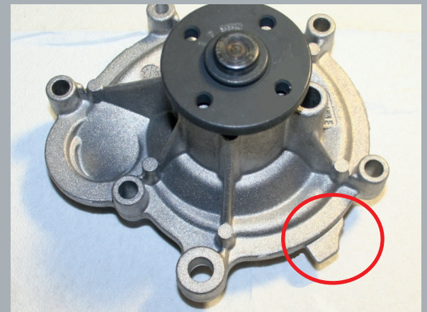
Bild 2: Wasserpumpe 65128
