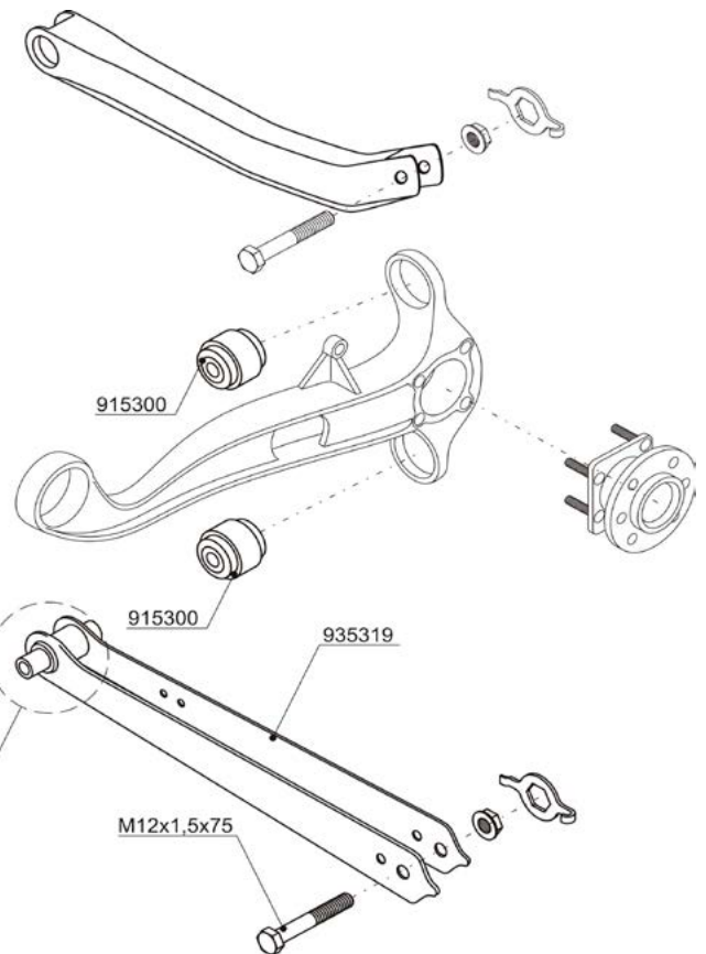
Εικόνα 1: Ράβδος Opel Vectra πίσω άξονα
