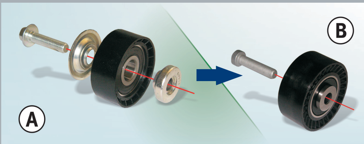
Umlenkrolle 55941, bisherige Ausführung (A) und neue Ausführung (B)
