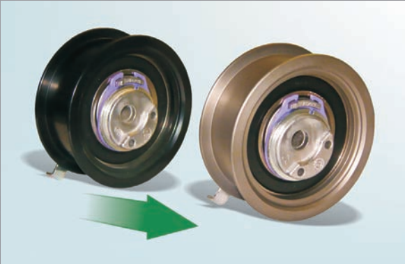
Bild 1: Verbesserte Beschichtung der Laufbahn - hier exemplarisch dargestellt an der Artikel-Nr. 55736
