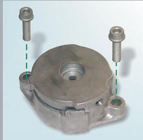
Bild 1: Ausführung mit zwei Schrauben M8x35
