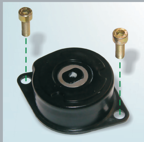
Bild 2: Ausführung mit zwei Schrauben M8x22
