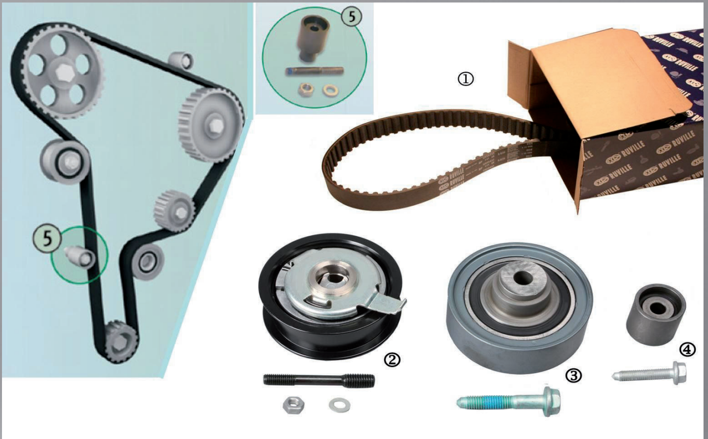
Bild 1: Triebschema 1.9 TDI/SDI und Packungsinhalt Kit 5549173/5549170
