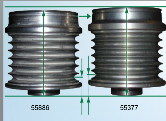
Bild 2: Unterscheidung der Generatorenfreiläufe 55886 (VALEO) und 55377 (DENSO)
