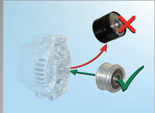
Bild 1: Artikelersetzung
