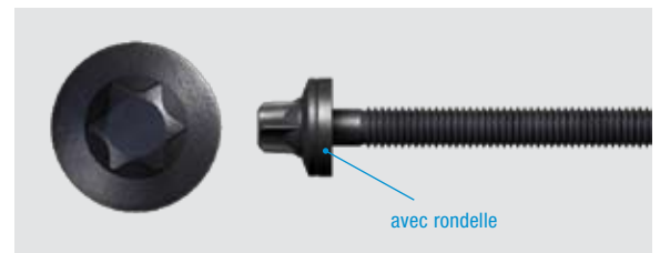
Illustration 1_Ancienne vis/vis remplacée avec rondelle (Réf. OE 607 926)
