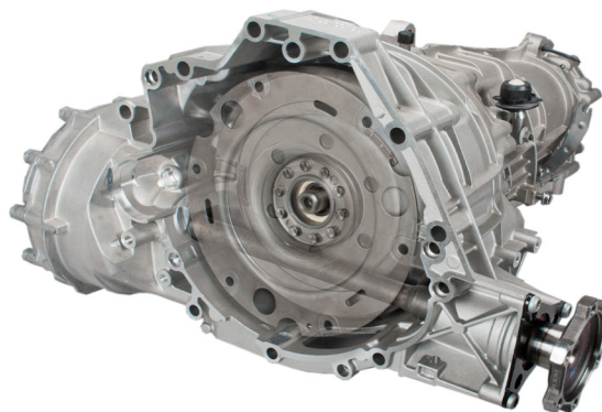
Bild 1: Framaxelns flänsaxel löper mellan drivplattan och dubbelmassavänghjulet
