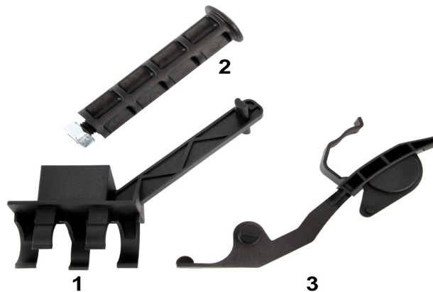
Bild 2: Verktögssett för montering med best. nr. 400 0537 10
