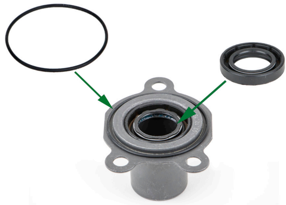
Douille de guidage avec joint torique et joint spi prémontés
