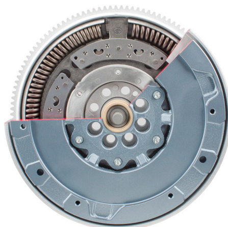
Снимка 1: Двумасов маховик с центробежна сила тип „махало”
