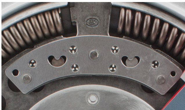
Снимка 2: Центробежна сила тип „махало”
