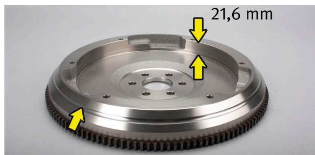
Billede 2: OE-nr. 93186460/5616016 med hulning i periferi; svinghjulets dybde: 21,6 mm
