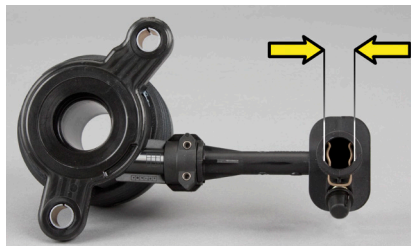
Снимка 2: Хидравлична връзка CSC на LuK 510 0097 10, 13,3 мм
