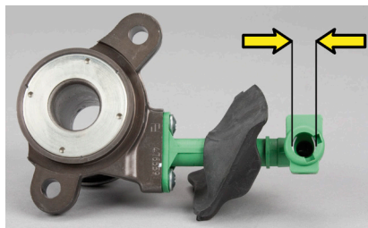
Снимка 4: Хидравлична връзка CSC на LuK 510 0137 10, 12,2 мм
