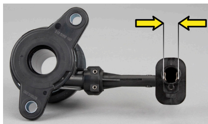
Снимка 1: Хидравлична връзка CSC на LuK 510 0090 10, 12,2 мм
