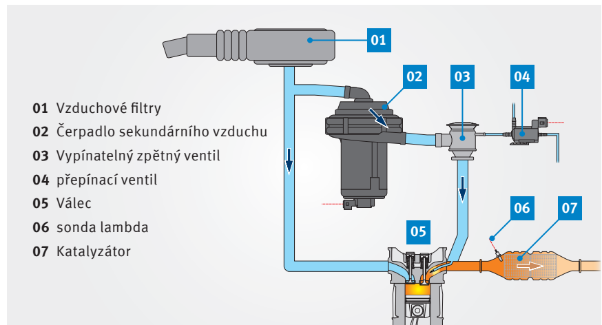
Princip vhánění sekundárního vzduchu (pneumatikky řízené)
