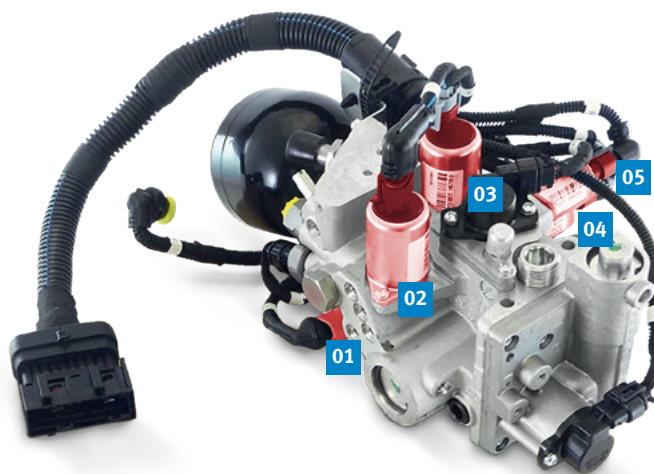
01–05 Пять управляющих клапанов (выделены красным) на секвентальной коробке передач Selespeed
