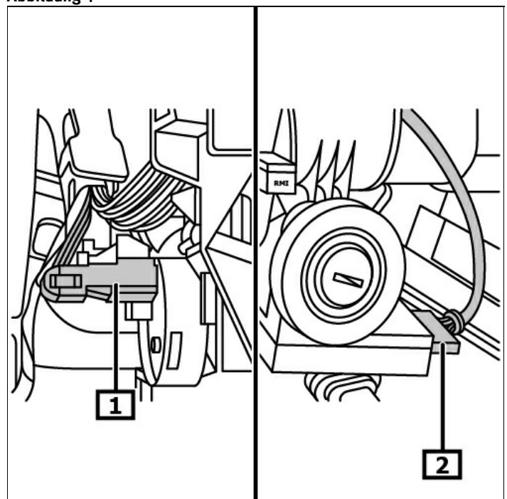
1 Elektr. Steckverbindung(en)
